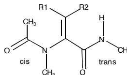
Rys. 1. Model N -metylodehydroaminokwasu z konfiguracją cis i trans wiązań amidowych
